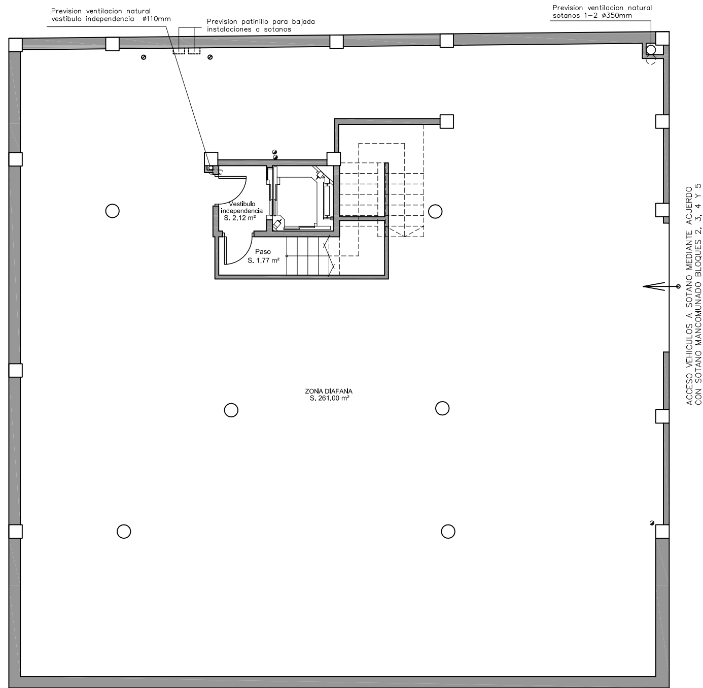
PLANTA SOTANO-1 E.-1:100
